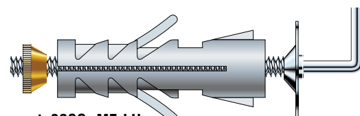
art. 92CO -ME-LU
